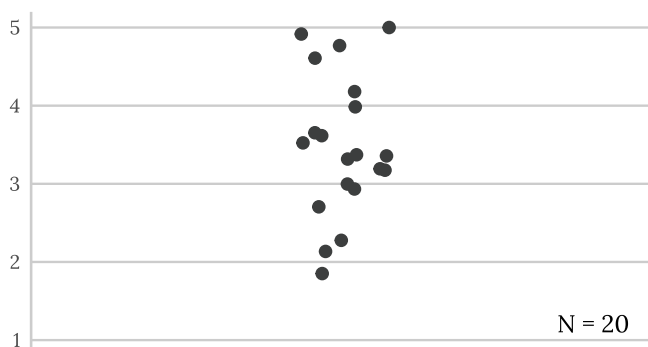
Abbildung 4: Individuelle Innovationsbereitschaft.
